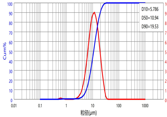
DXN-55 激光粒度分布曲线
