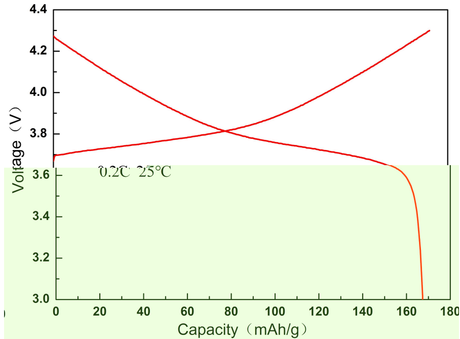
DXN-55 充放电曲线
